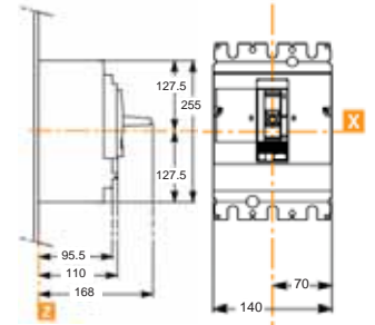
Kích thước EZC400/630
