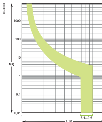
Đường cong hoạt động của thiết bị
