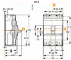
Kích thước EZC250
